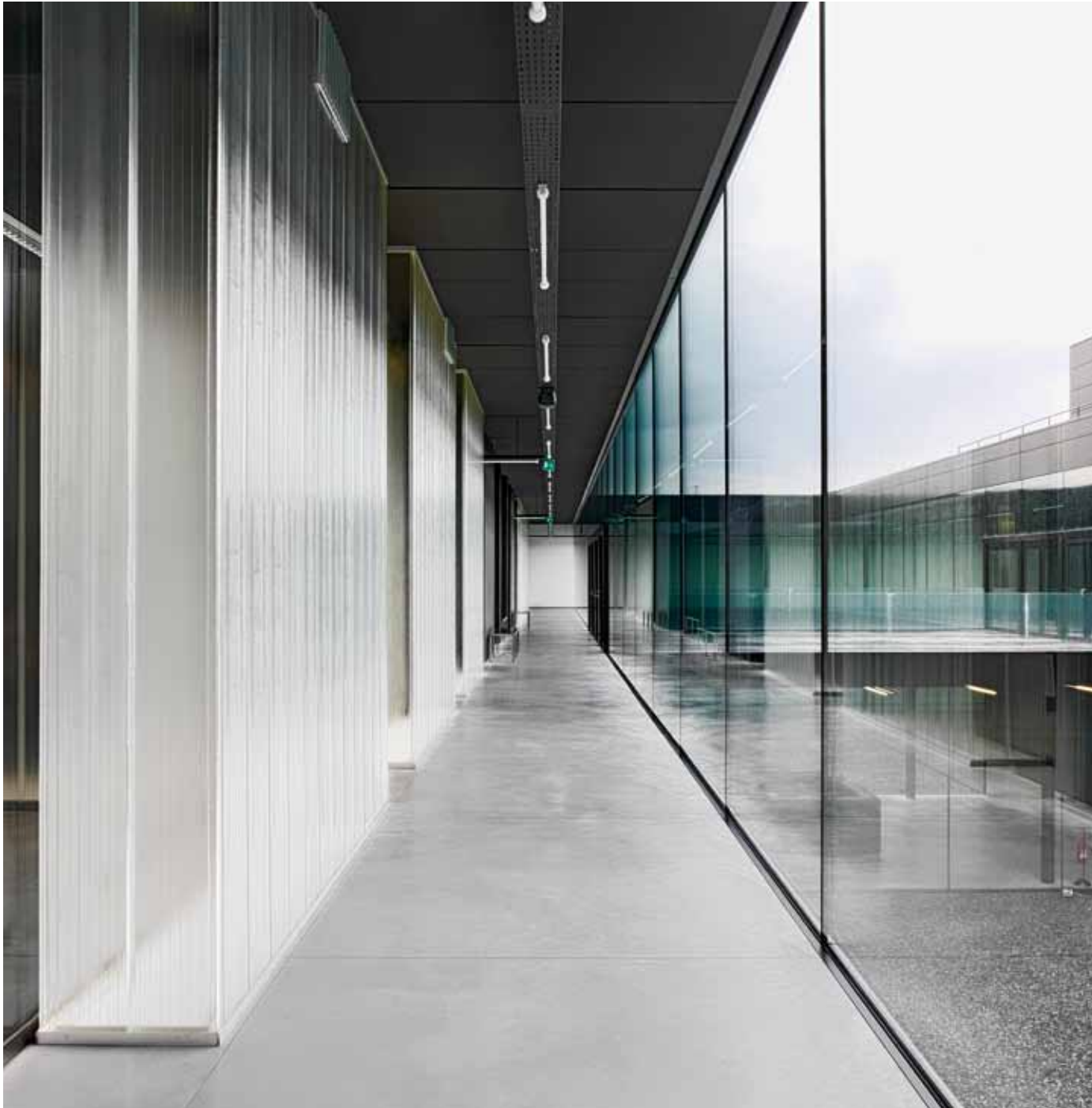
Veduta del corridoio al piano superiore: pareti in uglass armato con profilo in acciaio superiore ed inferiore.
